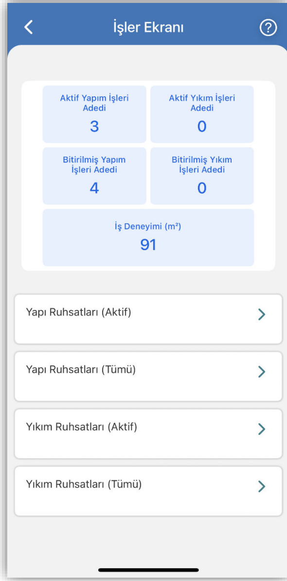
Şekil 20: İşler Ekranı
