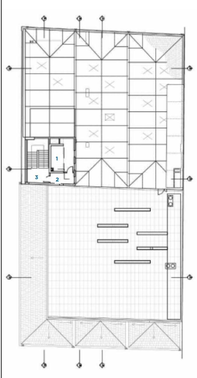
Üçüncü kat planı
