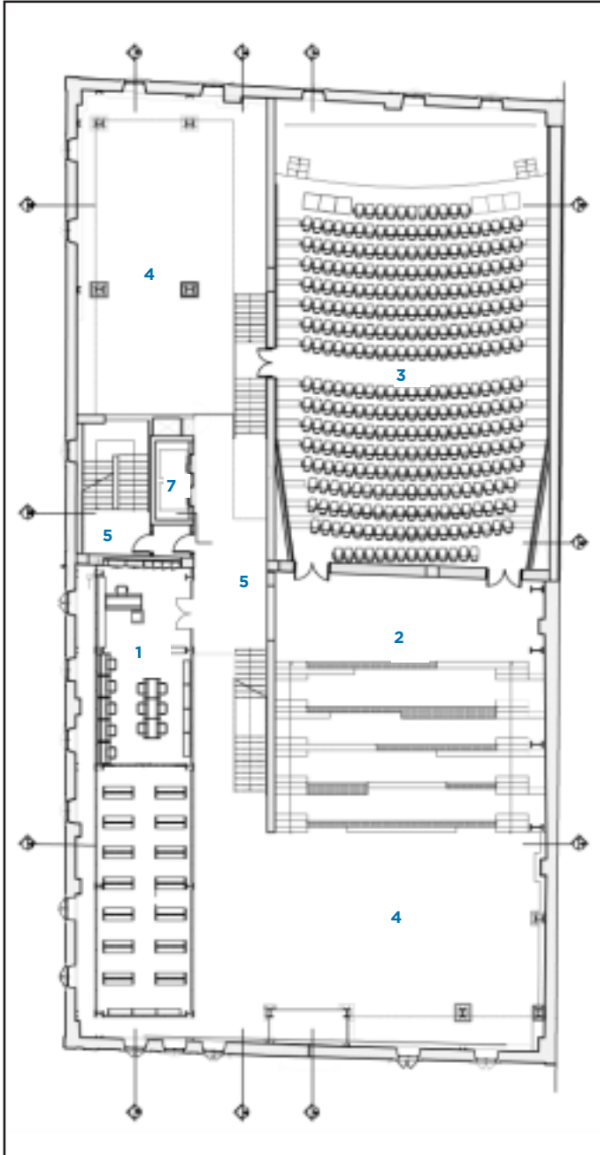
Ara kat planı
